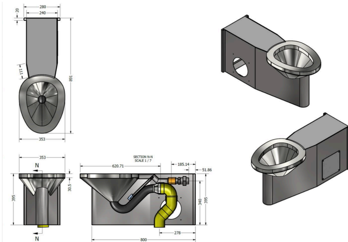
Figura 1. Vistas generales, vista superior y corte N-N (escala 1:7). Cotas en milímetros.
