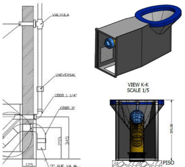
Figura 2. Detalle de instalación hidráulica y vista K-K (escala 1:5). Cotas en milímetros.
