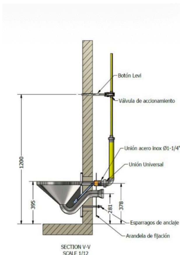
Figura 2. Corte V-V (escala 1:12): instalación en muro. Cotas en milímetros.
