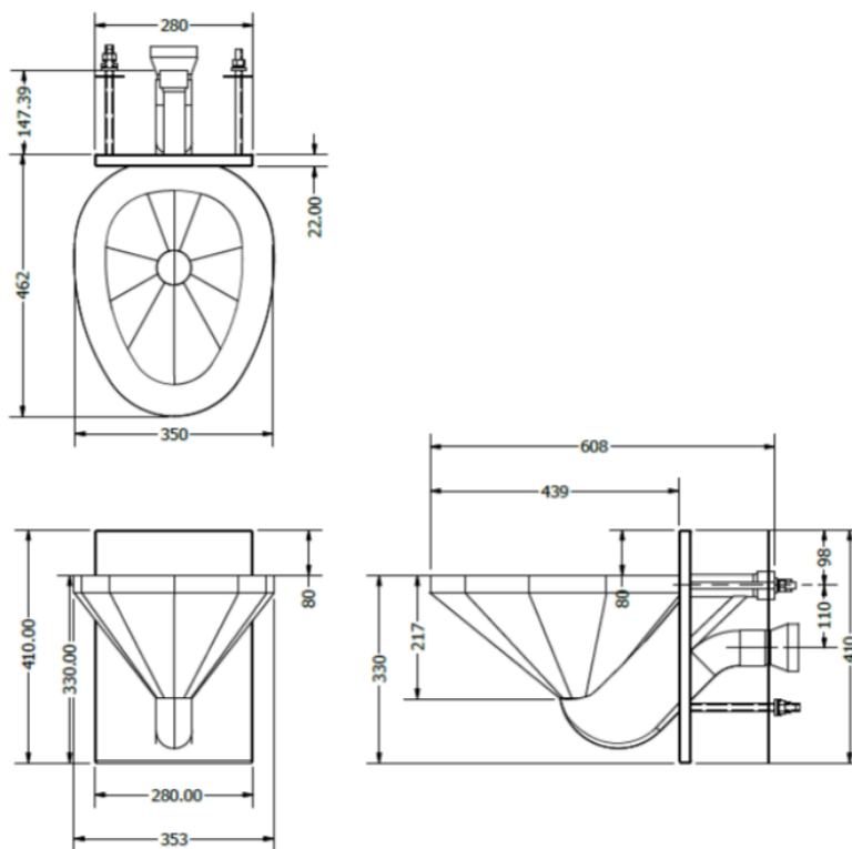
Figura 1. Vista superior, frontal y lateral. Cotas en milímetros.
