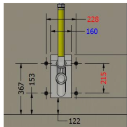
Figura 3. Vista posterior de conexiones y anclajes. Cotas en milímetros.
