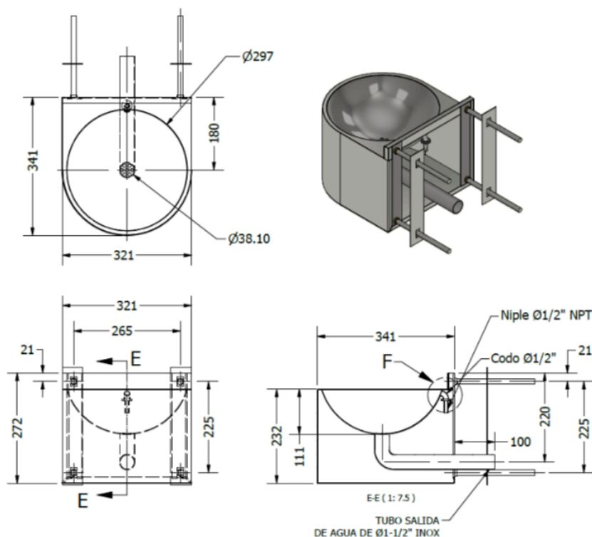
Figura 1. Planos y vista isométrica. Cotas en milímetros. Corte E-E (1:7,5).
